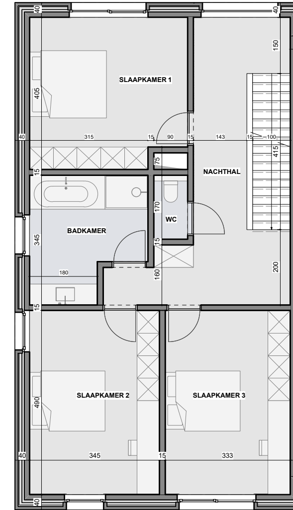
grondplan +01
