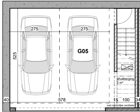
grondplan garage -01
